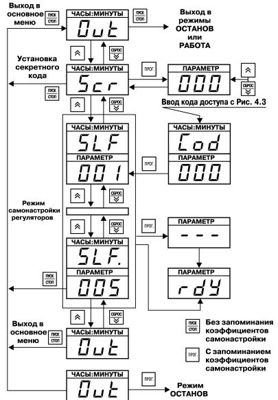
Рис. 4.5. Схема, поясняющая работу на уровне L3
