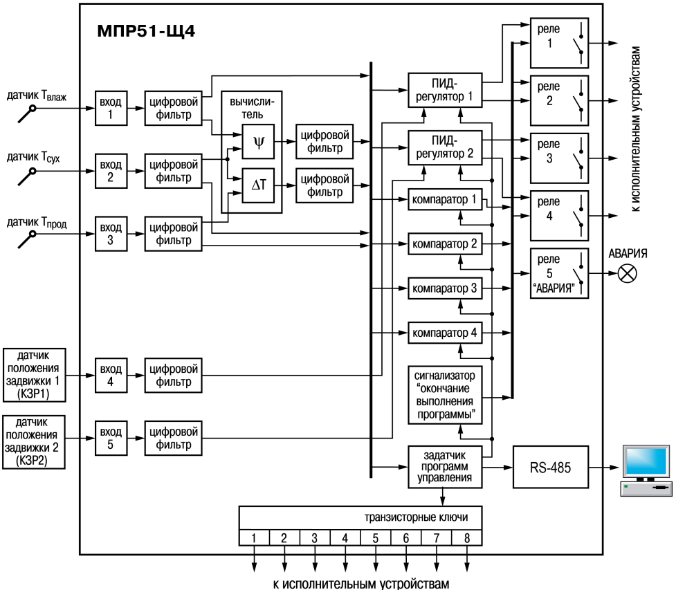
Рисунок 3.1. Структурная схема
