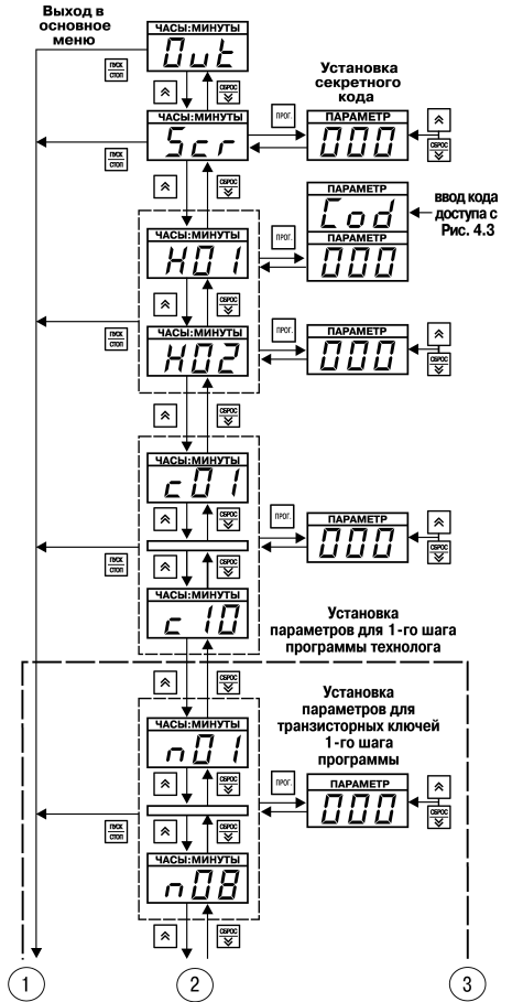
Рис. 4.4. Схема, поясняющая программирование на уровне L1
