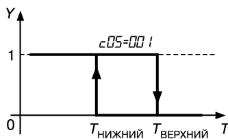
Рис. 3.15. Компаратор срабатывает по нижней уставке: Y = 1 - выходное реле замкнуто; Y = 0 - выходное реле разомкнуто
