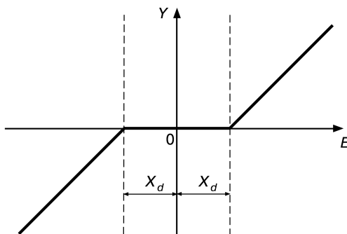
Рис. 3.13. Зона нечувствительности для исполнительного устройства типа "нагреватель - холодильник" или "задвигка"
