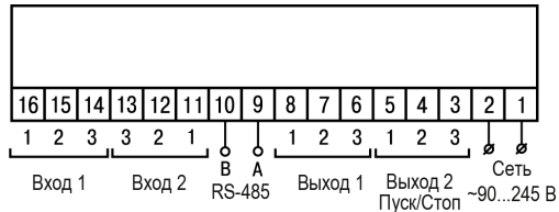
Рисунок 5.3 – Общая схема подключения TRM210-Н2
