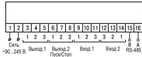
Рисунок 5.2 – Общая схема подключения TRM210-Н, -Щ1 и -Щ2
