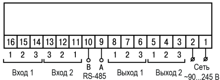
Рисунок 5.3 – Назначение контактов клеммника ТРМ212-Н2
