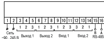
Рисунок 5.2 – Назначение контактов клеммника ТРМ202-Н, -Щ1 и -Щ2
