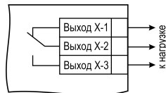
Рисунок 5.12 – Схема подключения нагрузки к ВУ типа P
