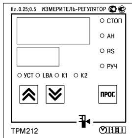
Рисунок 6.2 – Лицевая панель прибора для корпусов: 1) настенного Н и щитового Щ1 крепления, 2) щитового Щ2, 3) настенного Н2
