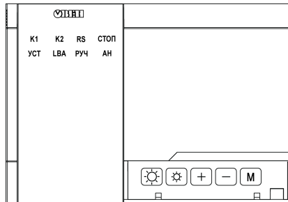
Рисунок 6.2 – Лицевая панель прибора для корпусов: 1) настенного Н и щитового Щ1 крепления, 2) щитового Щ2, 3) настенного Н2
