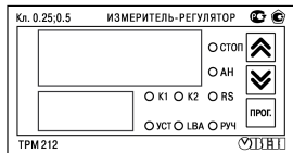
Рисунок 6.2 – Лицевая панель прибора для корпусов: 1) настенного Н и щитового Щ1 крепления, 2) щитового Щ2, 3) настенного Н2
