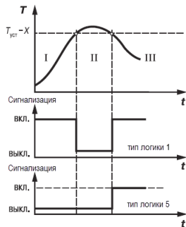
Рисунок 7.10 – Срабатывание сигнализации в системе нагревания
