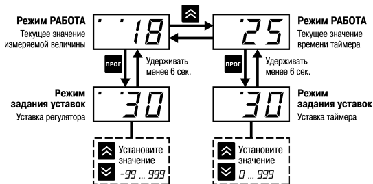
Рисунок 7.1 – Схема задания уставок регулятора и таймера
