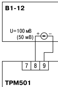
Рисунок 8.4 – Схема подключения
