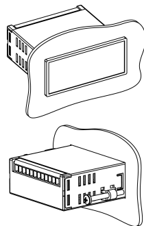
Рисунок 4.1 – Установка прибора щитового крепления
