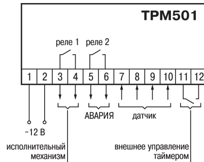
Рисунок 5.1 – Описание клеммника
