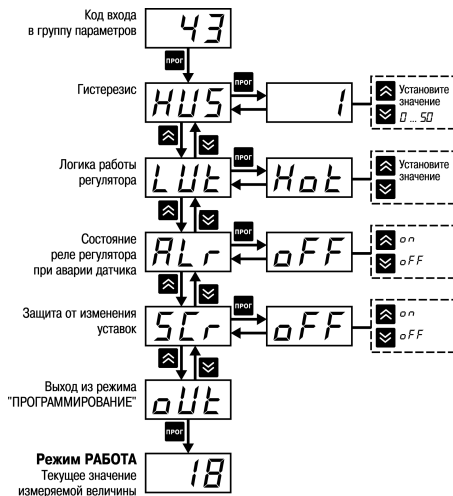
Рисунок 7.5 – Алгоритм настройки параметров регулятора
